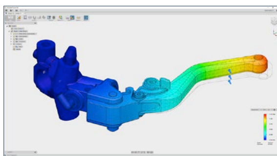
線形静解析を表示している例
